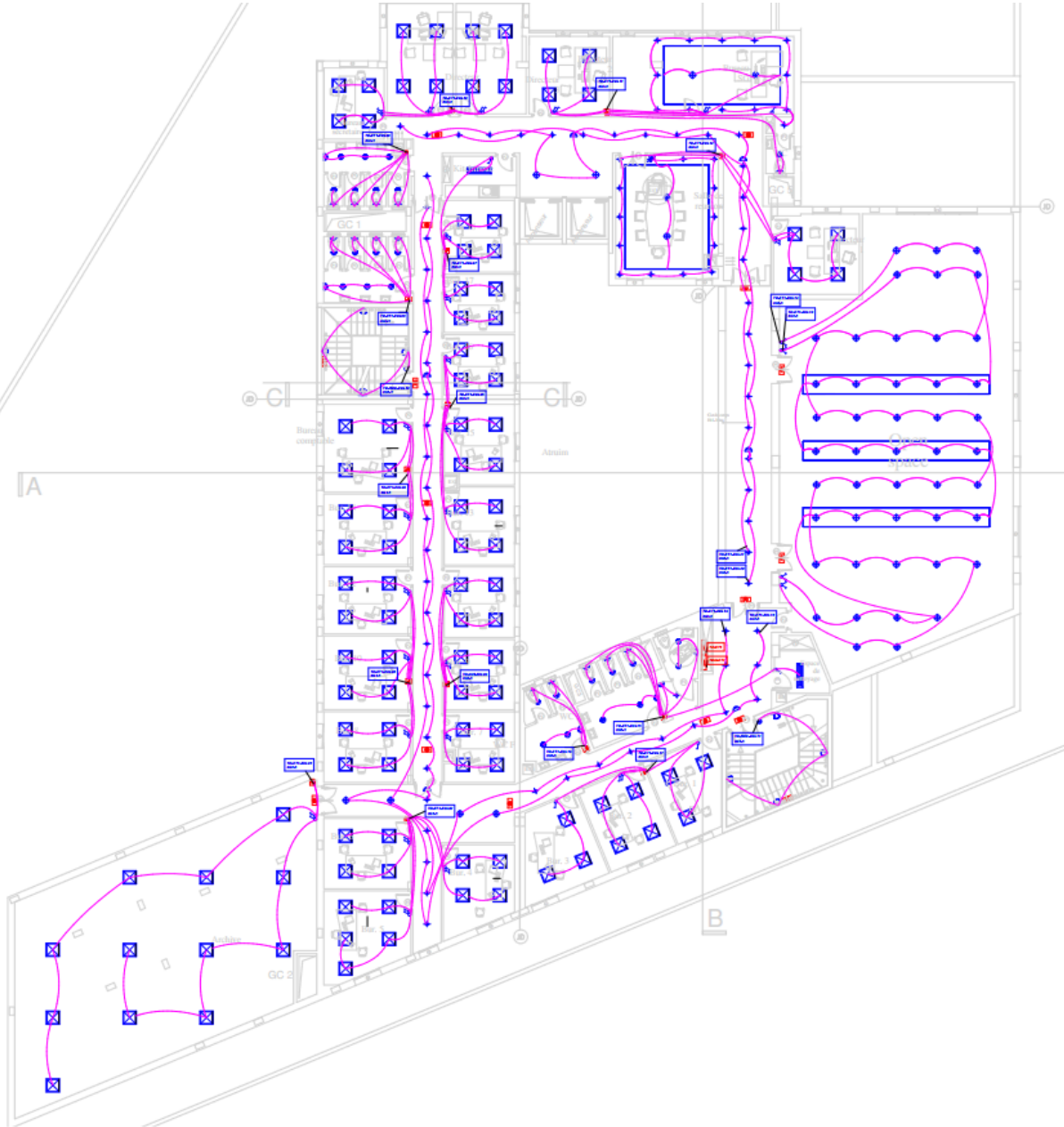
PLAN ECL ETAGE 1 ET ETAGE 2
