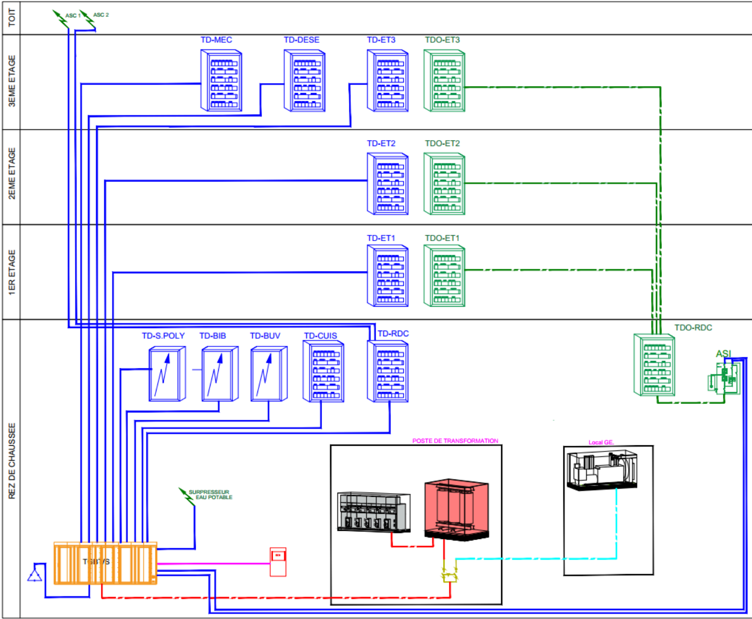
SYNOPTIQUE COURANT FORT
