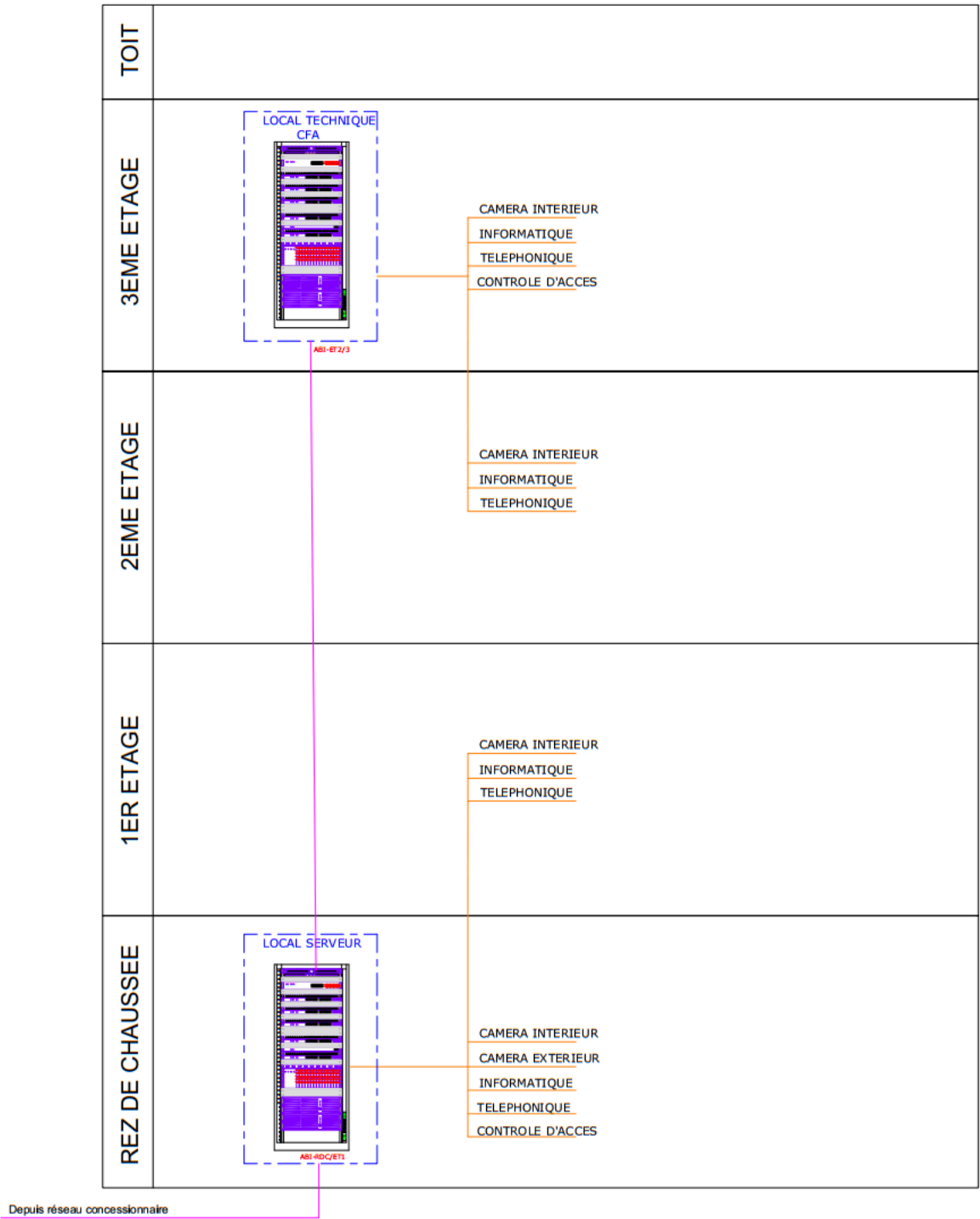
SYNOPTIQUE COURANT FAIBLE
