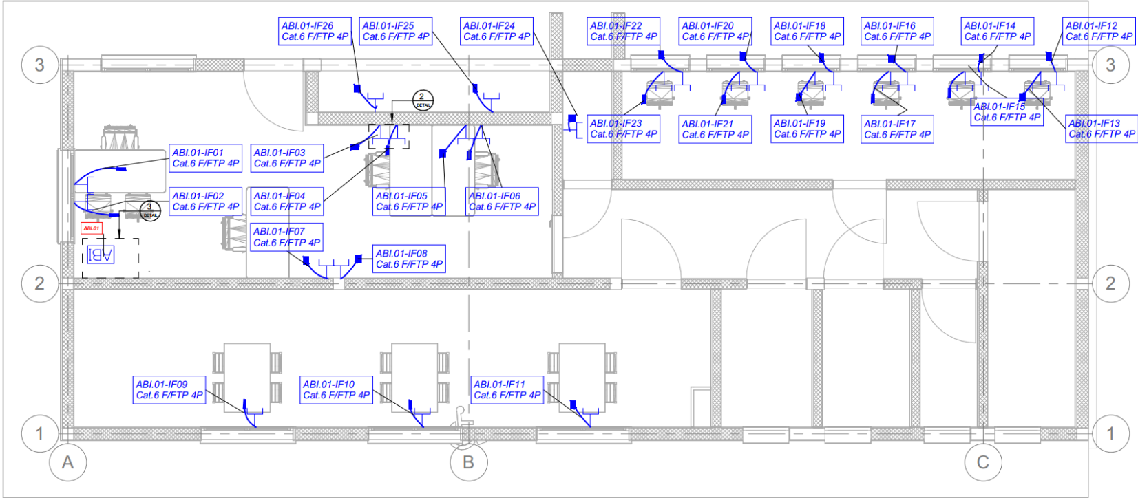
1 PLAN DE PRECABLAGE INFORMATIQUE-RDC 1 : 50
