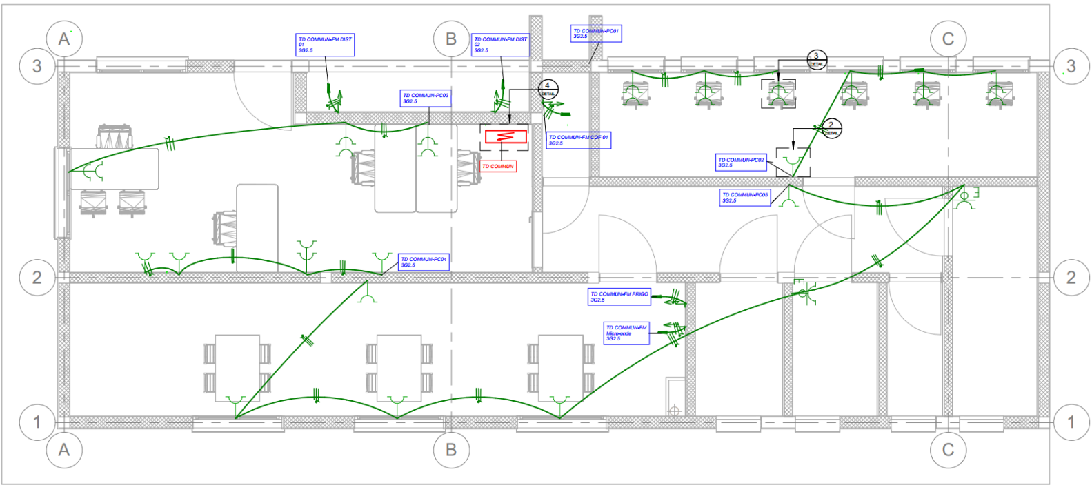
1 Plan prise courant et alimentation divers-RDC 1 : 50
