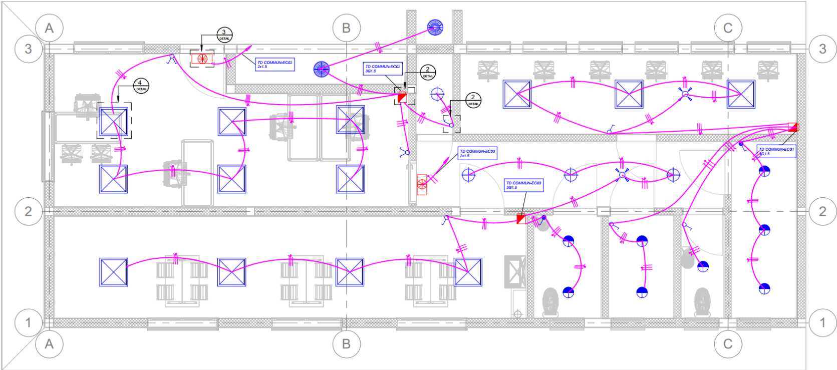
1 PLAN ECLAIRAGE ET ECLAIRAGE DE SECURITE_RDC 1 : 50
