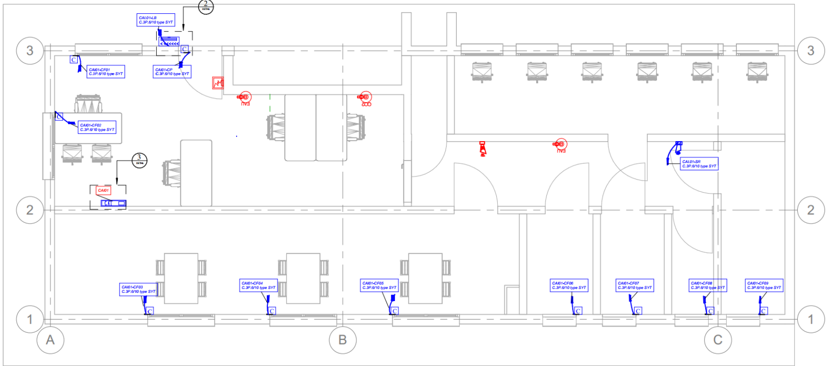
1 PLANE DE SYSTEME DE SECURITE_RDC Y COMPRIS LES EXTINCTEUR 1 : 50
